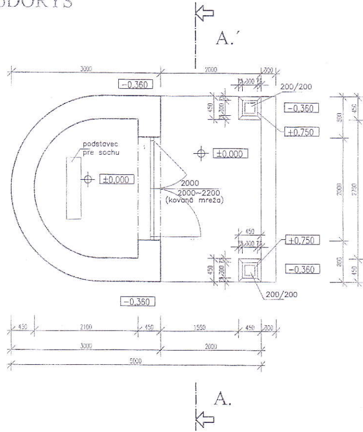
PŮDORYS
